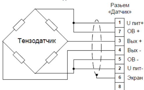
Схема подключения тензодатчика
