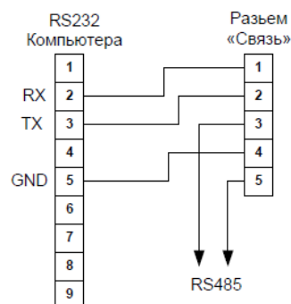
Схема распайки кабеля связи
